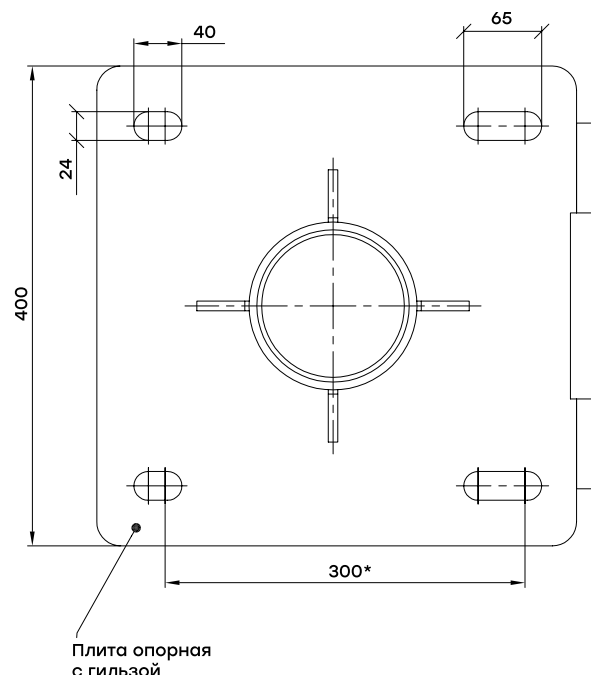
Схема основания (для молниеотводов ММСПА от 15 до 25 м включительно и ММСАА высотой от 15 м до 22 м включительно)
